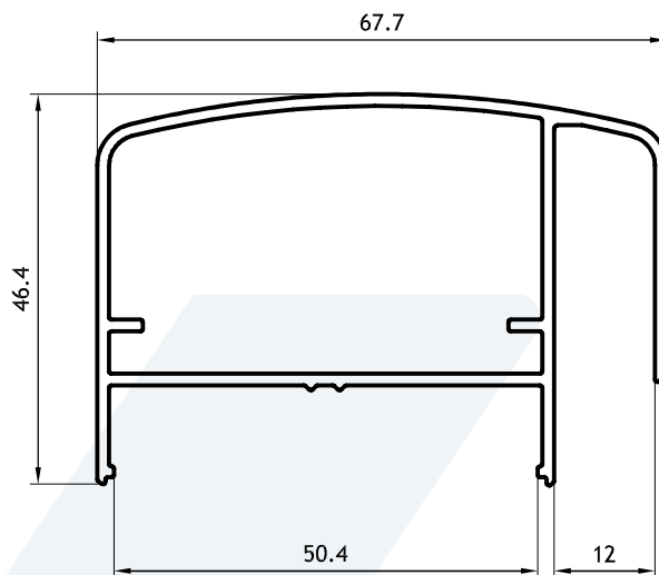
Pasamanos Rectangular 0,930 kg/m 09201 Barras de 6.20m
