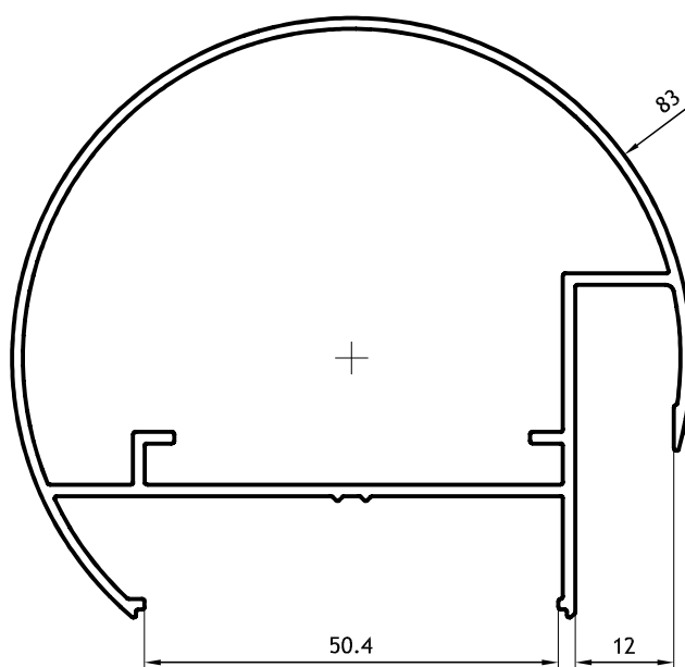
Pasamanos Redondo 1,160 kg/m 09200 Barras de 6.20m
