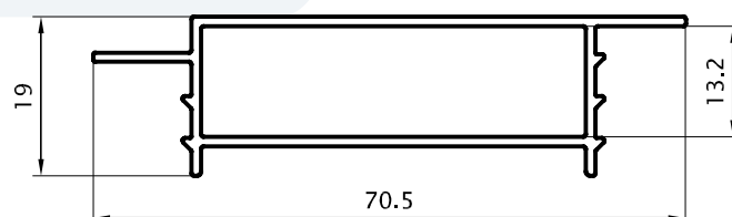
Premarco 0,494 kg/m 00147 (Barras de 6.05m)
