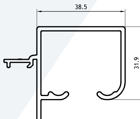
Guía Marco Superior Puerta Libro 0,730 kg/m 02872 Barras de 6.05m 6 Barras por Paquete
