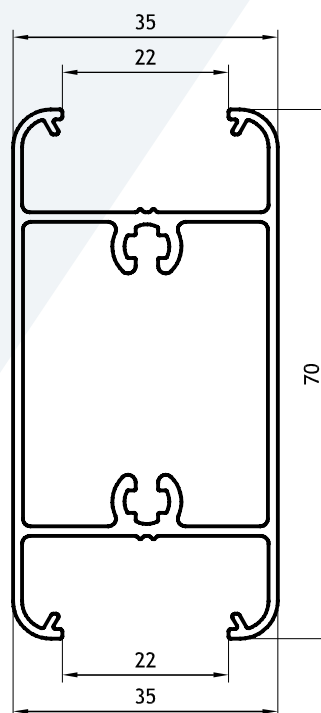
Travesaño 70 mm DVH 0,961 kg/m 02882 Barras de 6.05m 18 Barras por Paquete
