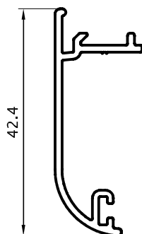
Tapajuntas 0,312 kg/m 09012 (Barras de 6.05m)
