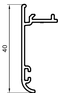
Tapajuntas 0,251 kg/m 09011 (Barras de 6.05m)
