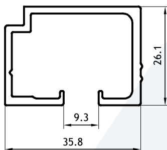
Guía Marco Puerta Libro 0,580 kg/m 02871 Barras de 6.05m 6 Barras por Paquete
