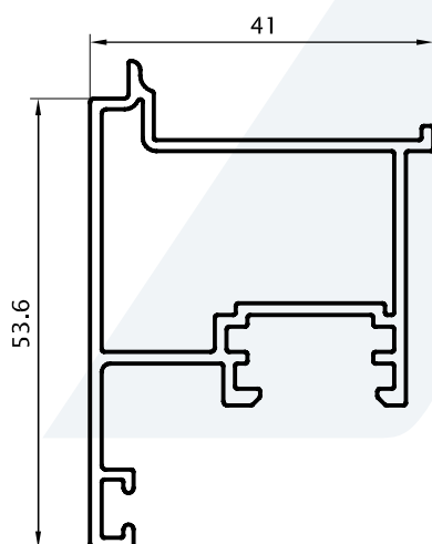
Encuentro Hojas de Abrir 0,754 kg/m 02853 (Barras de 6.05m)
