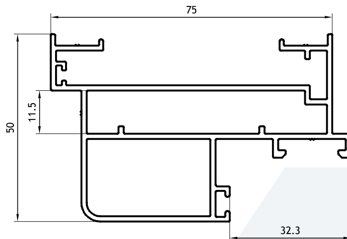
Marco Puerta Libro 1,292 kg/m 02870 Barras de 6.05m 4 Barras por Paquete
