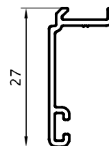
Tapajuntas 0,148 kg/m 09013 (Barras de 6.05m)
